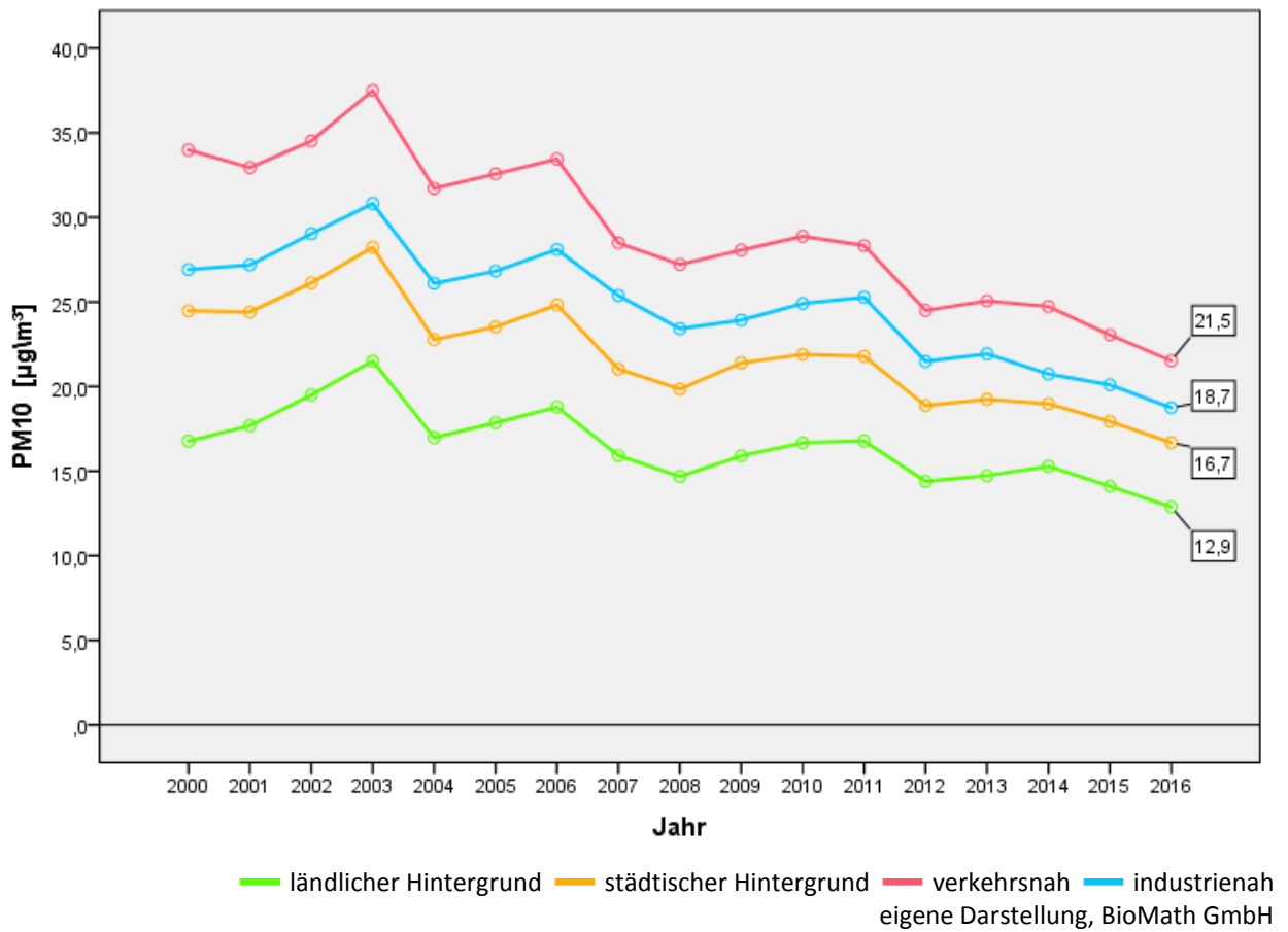
Abbildung 7: Jahresmittelwertzeitreihen des Modells für PM10
