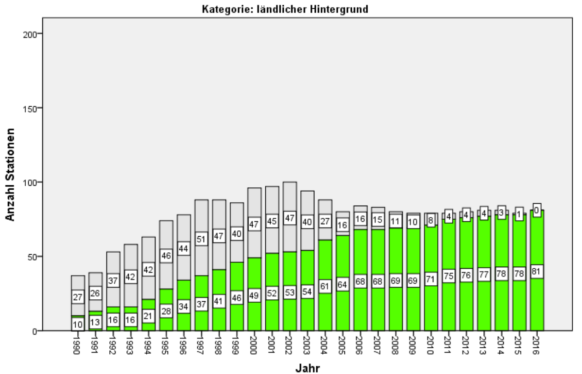
■ durchgängig messend bis 2016 ■ nicht durchgängig messend bis 2016 eigene Darstellung, BioMath GmbH
