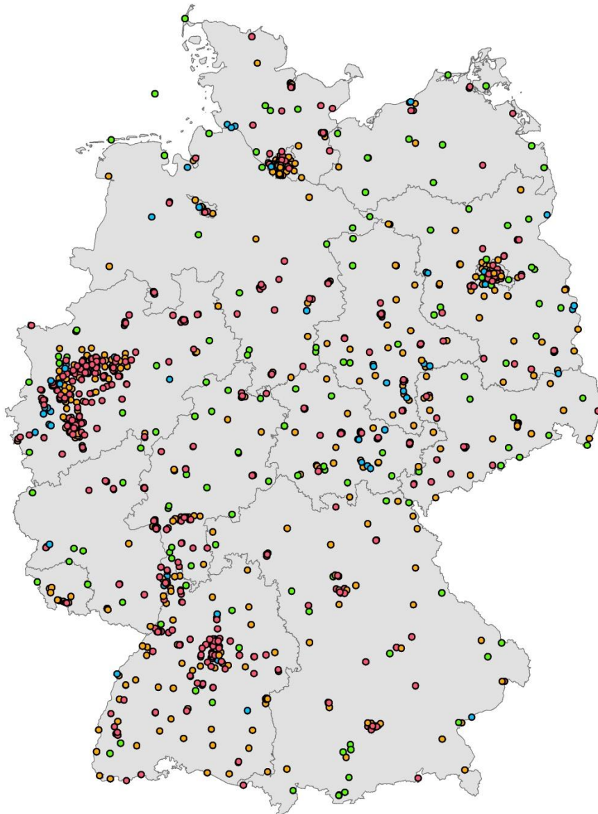
Abbildung 2: NO2 - Karte mit allen Messstationen von 1990-2016
