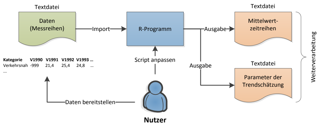
Abbildung 8: Verarbeitungsschema R-Programm
