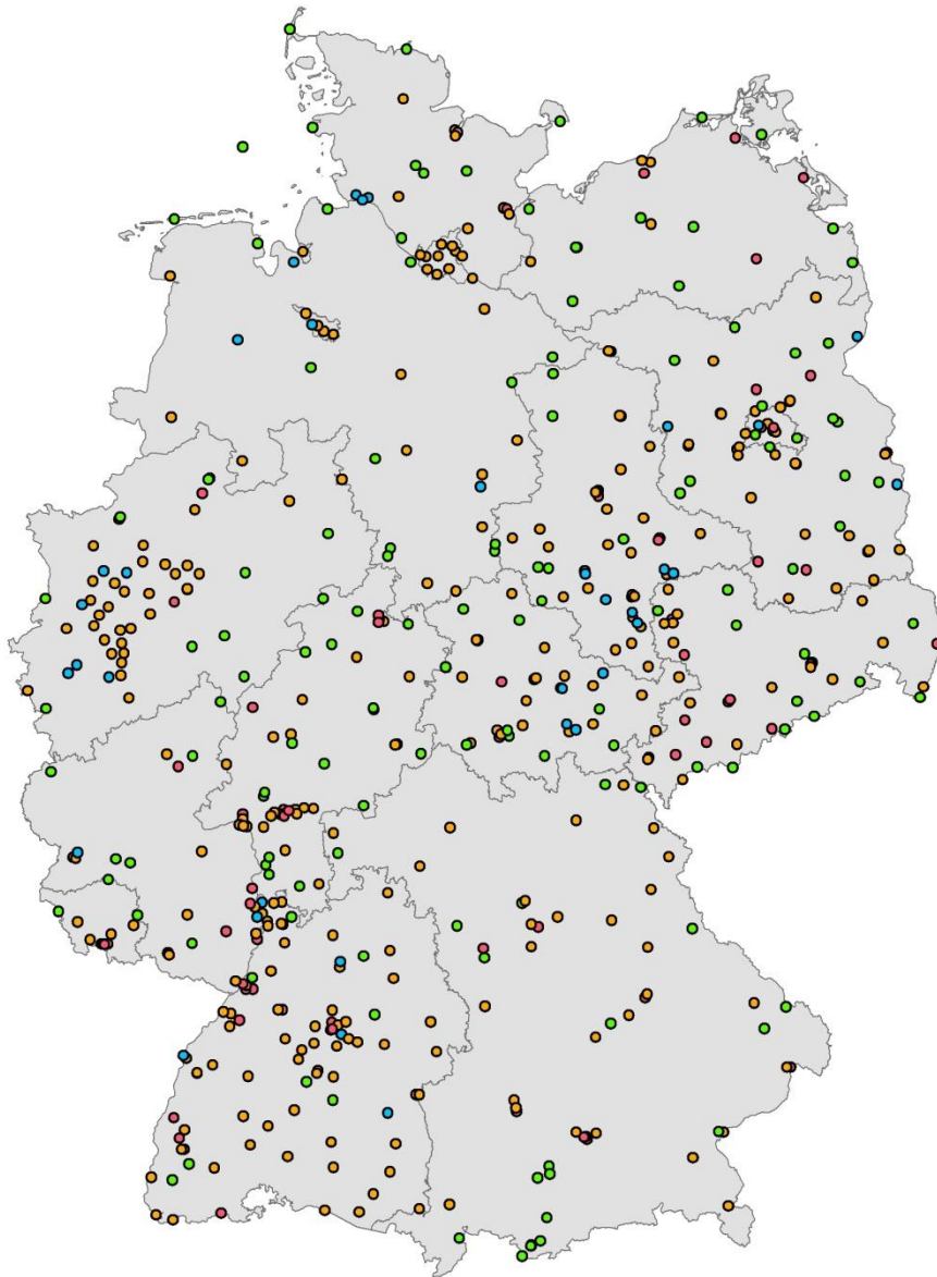
Abbildung 1: Ozon - Karte mit allen Messstationen von 1990-2016
