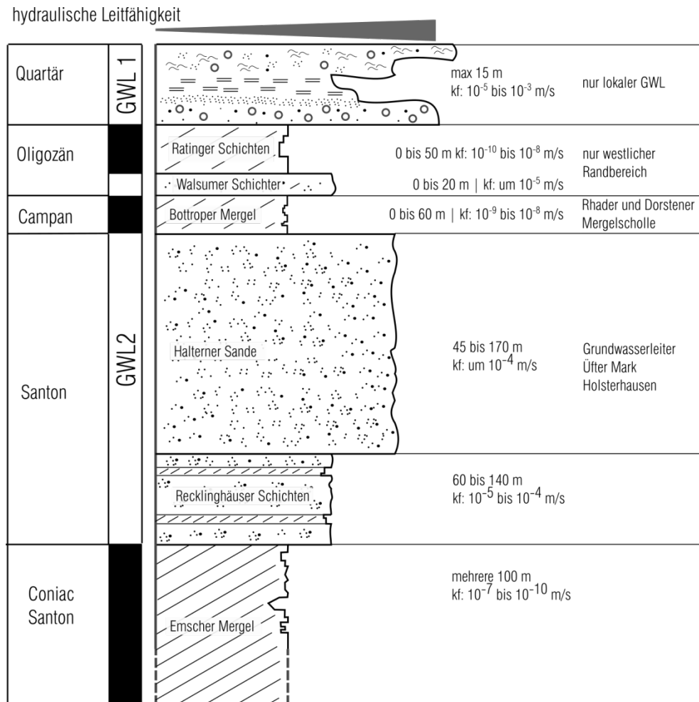
Abbildung 21: Schematische Darstellung der Schichtenfolge im Wassergewinnungsgebiet Holsterhausen/Üfter Mark
