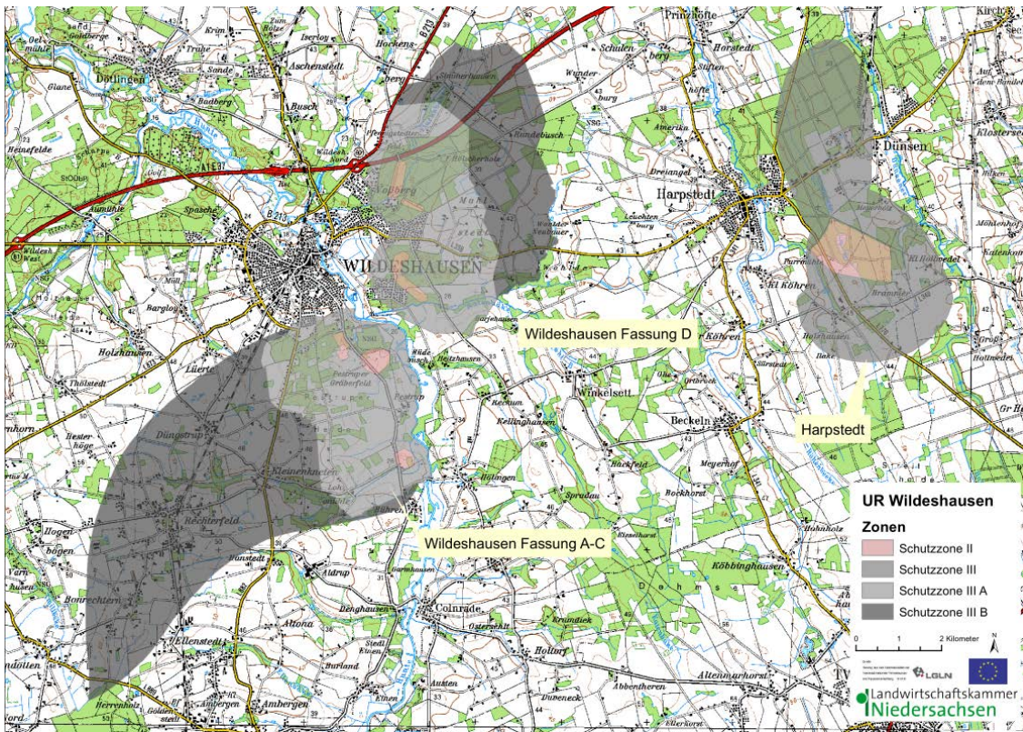
Abbildung 71: Geografische Karte der TGG der Kooperation OOWV, Wildeshausen
