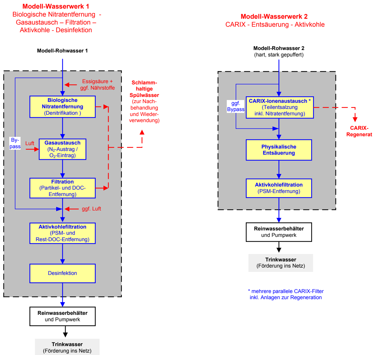
Abbildung 30: Verfahrensschemata für die Modellwasserwerke 1 und 2
