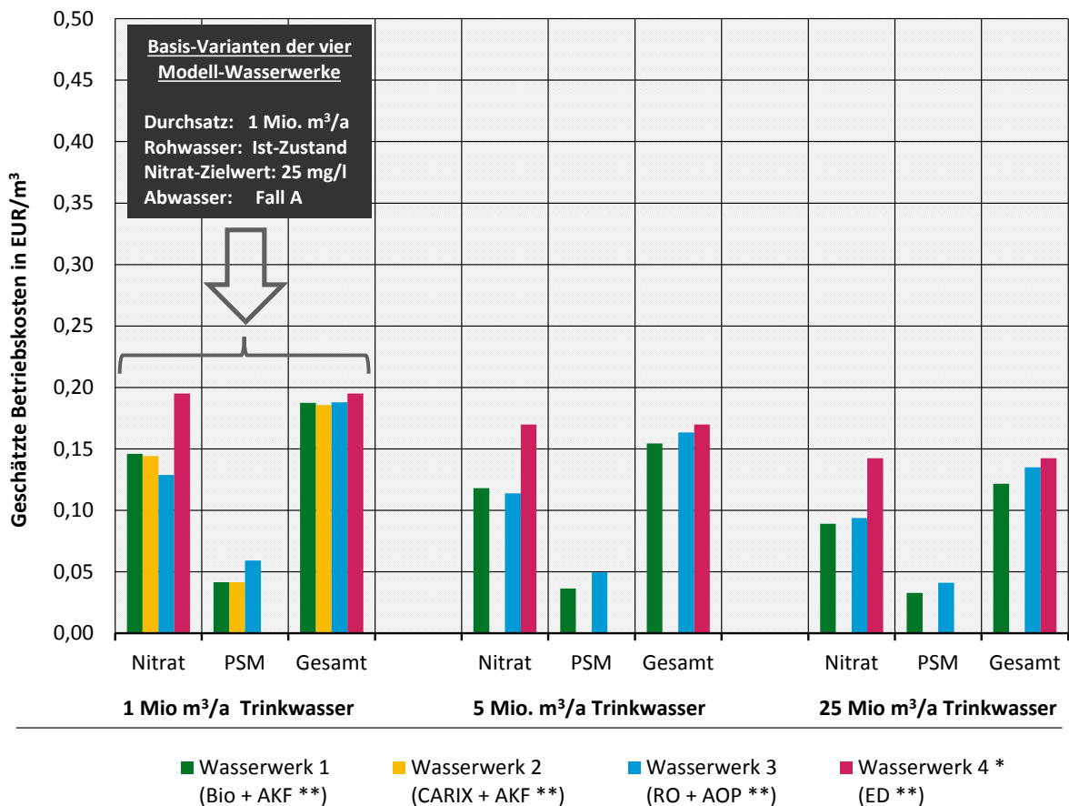
Abbildung 34: Spezifische Betriebskosten für verschiedene Wasserwerksgrößen
