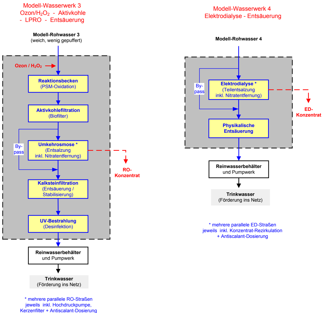
Abbildung 31: Verfahrensschemata für die Modellwasserwerke 3 und 4
