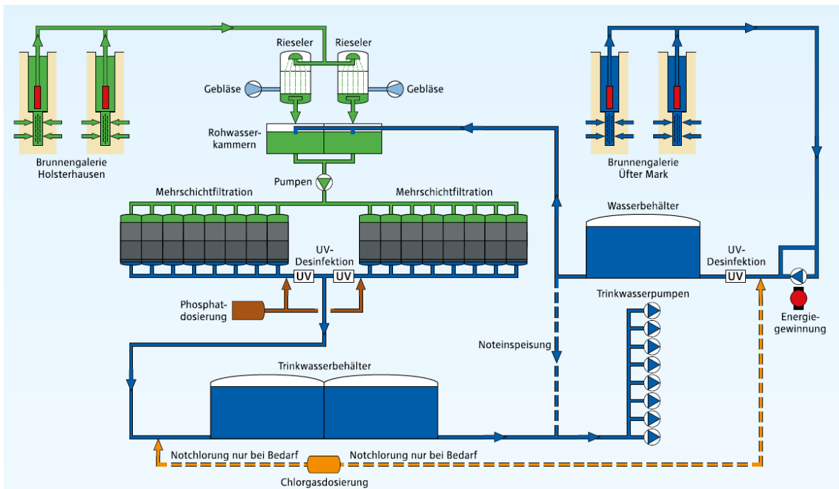
Abbildung 29: Schematische Darstellung der aktuellen Fördersituation des Wasserwerkes Dorsten Holsterhausen
