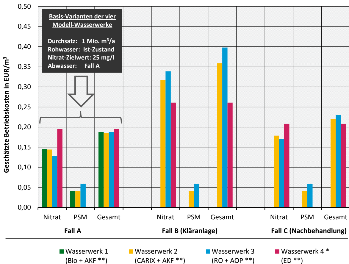
Abbildung 36: Spezifische Betriebskosten für verschiedene Arten der Abwasserentsorgung
