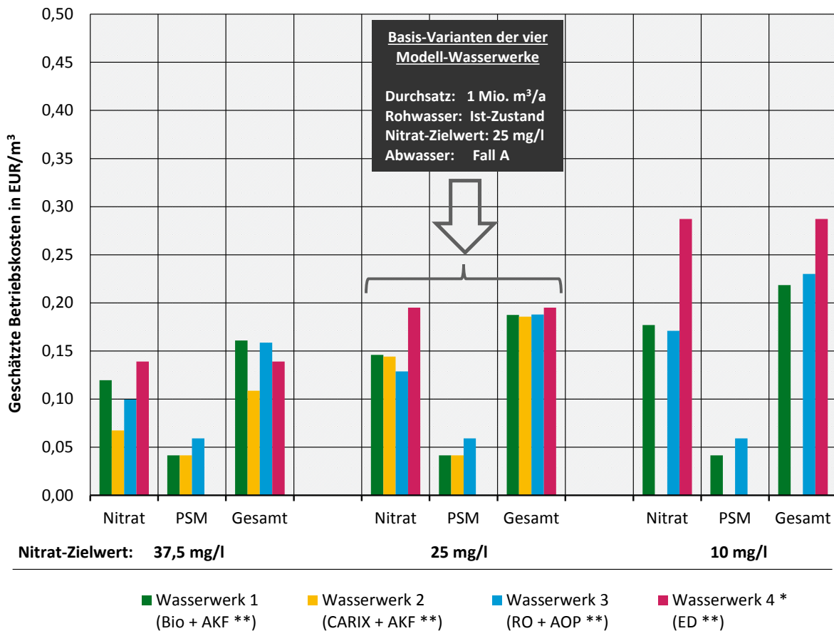
Abbildung 35: Spezifische Betriebskosten für verschiedene Nitrat-Zielwerte (Q = 1 Mio. m 3 /a)
