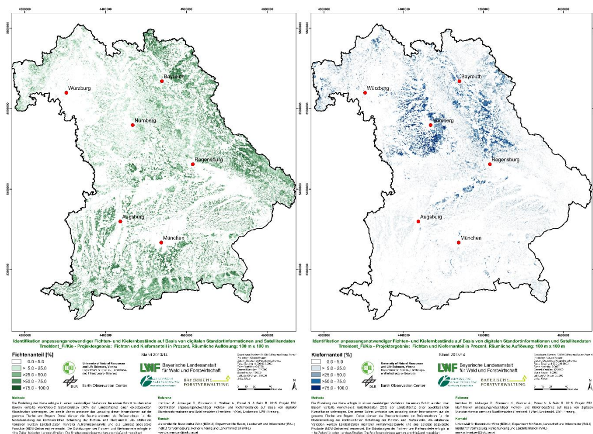
Abbildung 4 Fichten und Kiefernverbreitungskarten von Bayern basierend auf multi-temporalen Landsat Daten
