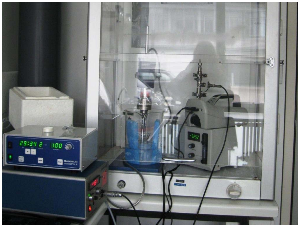
Abbildung 6: Aufbau der Messgeräte beim Homogenisieren mittels Ultraschall im Laborabzug
